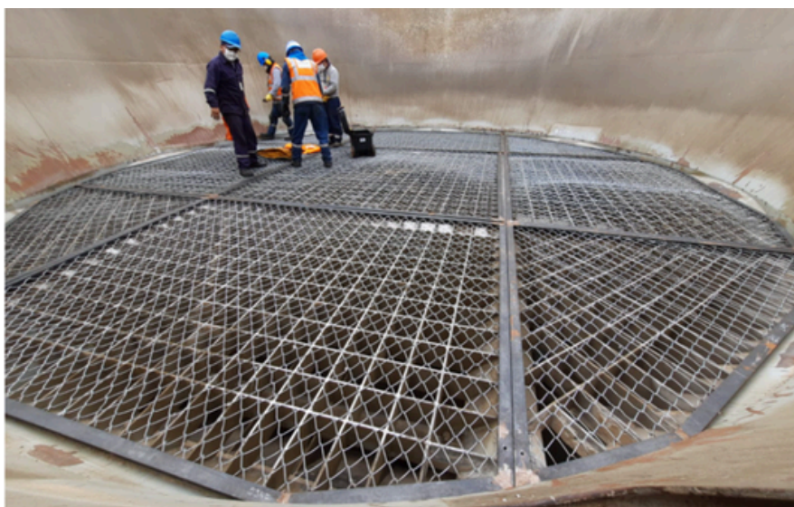
DISEÑO Y FABRICACIÓN DE MALLA FILTRO PARA GRANOS
